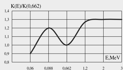
Типовая энергетическая зависимость чувствительности прибора относительно энергии 662 кэВ гамма-излучения ^{137}\text{Cs}
